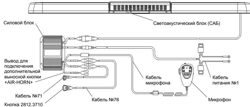
Рисунок 1.1 - Общий вид СГУ
